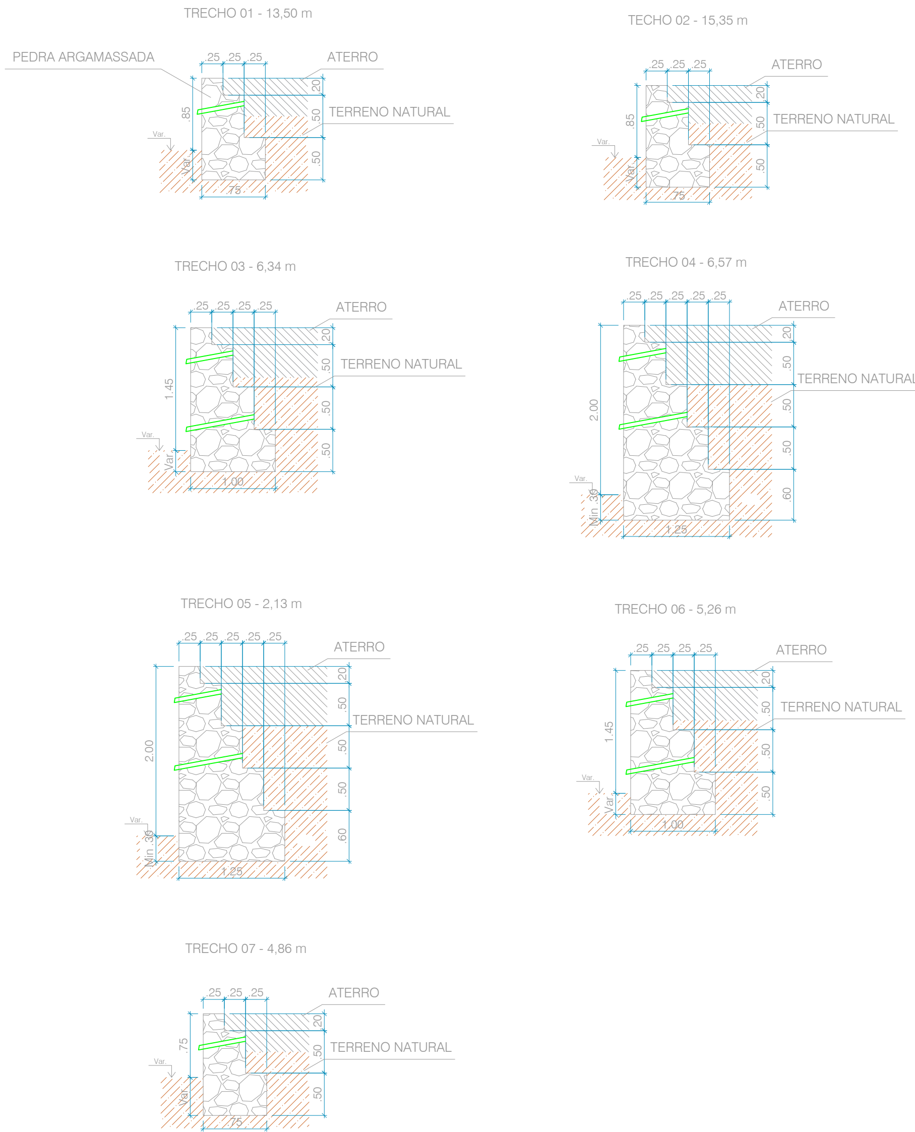
SEÇÃO TIPO
